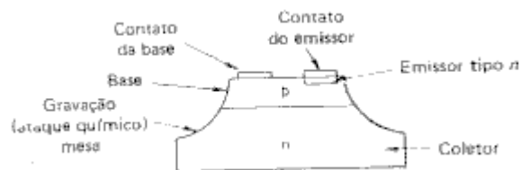
Figura 8.41 Serão transversal do transistor mesa
