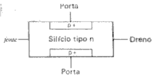
Figura 8.49 Estrutura esquemática do transistor de junção por efeito de campo
