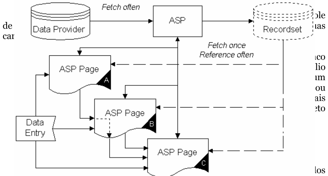
Figura 6: ADO e ASP.
