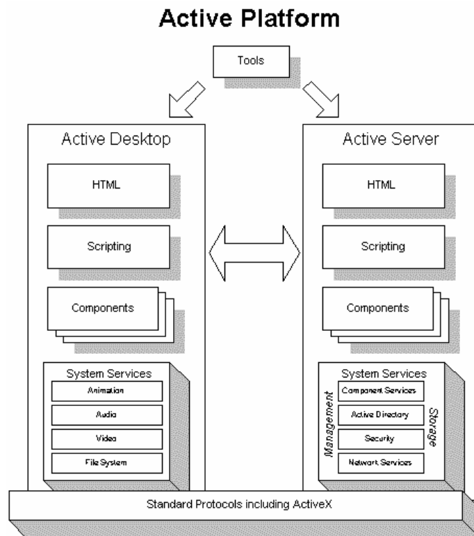
Figura 1: Visão da Microsoft sobre o Active Platform.
