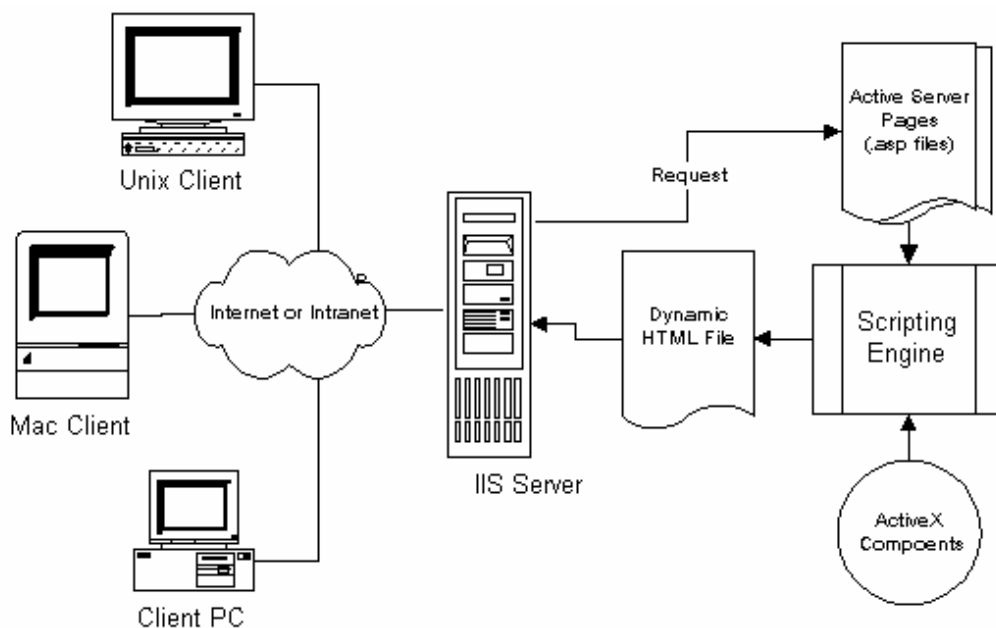
Figura 4: Funcionamento do ASP.
