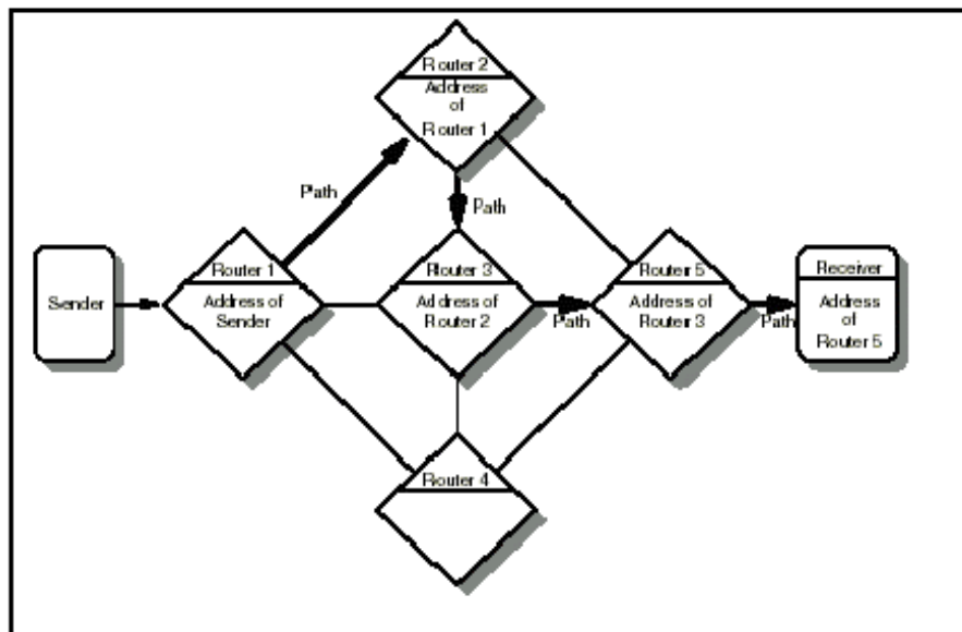
Figura 3.5 – Processo de definição de um caminho RSVP
