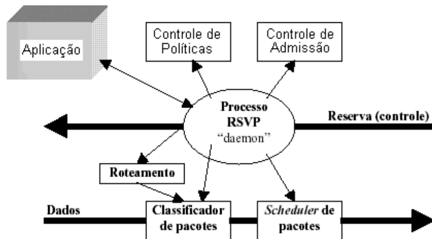
Figura 3.2 – Módulos necessários em uma implantação RSVP.
