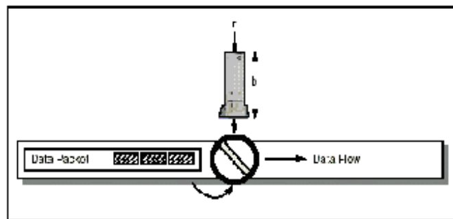
Figura 3.4 – “Token Bucket” (balde de fichas)
