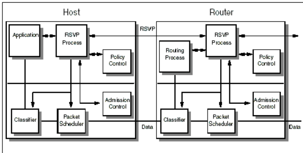
Figura 3.3 – Modelo de Serviços Integrados.
