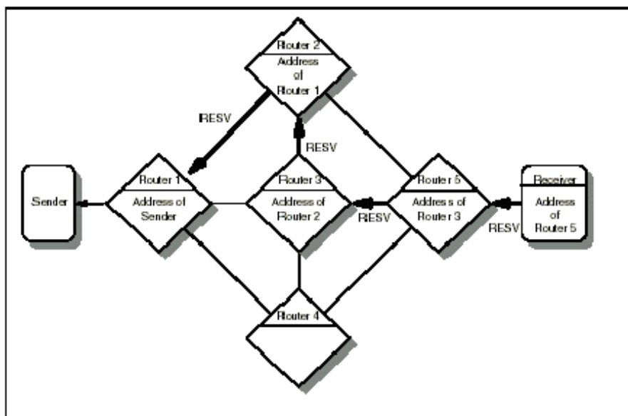
Figura 3.6 – Fluxo de mensagens de requisição de reserva RSVP
