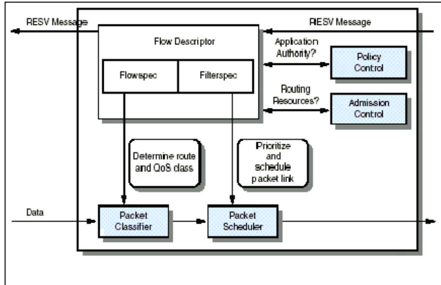
Figura 3.7 – Processo de reserva RSVP
