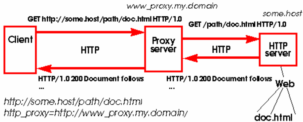
Figura 3: Uma trasação HTTP com proxy. O cliente faz uma requisição ao proxy usando HTTP mas especificando toda a URL; o proxy se conecta ao servidor remoto e pede o recurso relativo àquele servidor sem especificar protocolo ou o nome do servidor na URL
