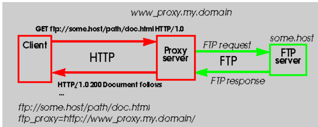
Figura 4: Trasação FTP com proxy. O cliente faz a requisição ao proxy usando HTTP (embora o recurso seja um FTP). O proxy analisa a URL recebida e percebe que deve abrir uma conexão FTP. O resultado (o arquivo, no caso) é enviado para o cliente usando HTTP
